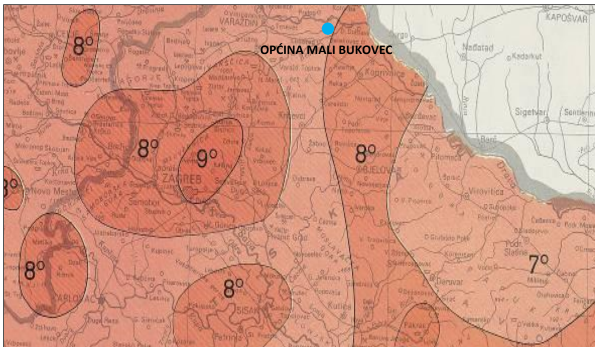
Slika 1. Seizmološka karta za povratni period od 500 godina
