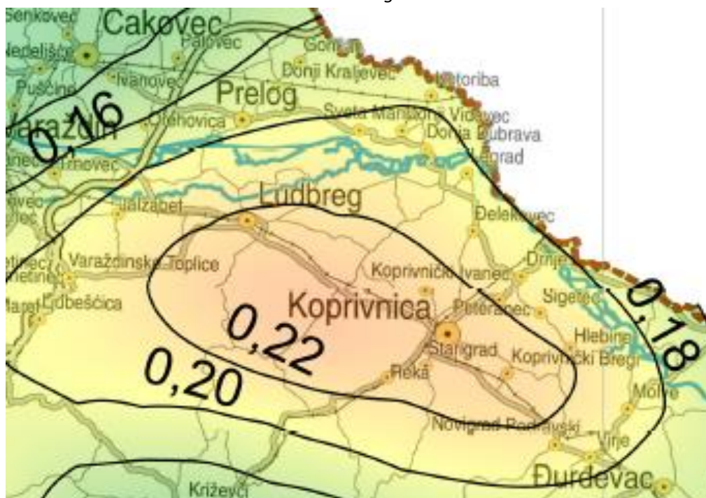
Slika 3. Vršna ubrzanja tla uzrokovana potresima za područje Općine Mali Bukovec, za povratni period 475 godina
